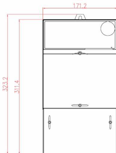
Abb. 1: Frontansicht
