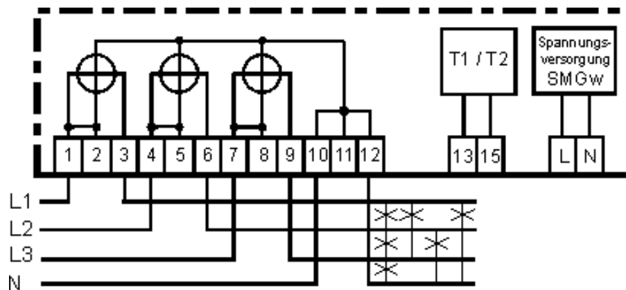
Abb. 5: Schaltbeispiel
